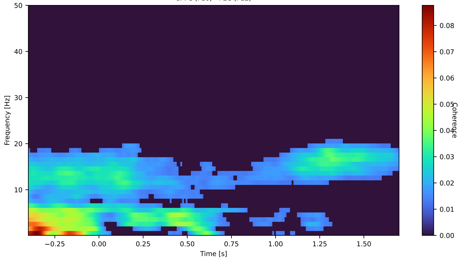
dPFC (F10) - PEC (P12)
